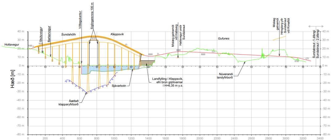
↑ 8 Sundabrá, langsnið.
