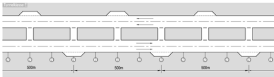
Figur 4.5 Tunnelklasse E, havarinisjer, nødstasjoner og tverrförbindelser
